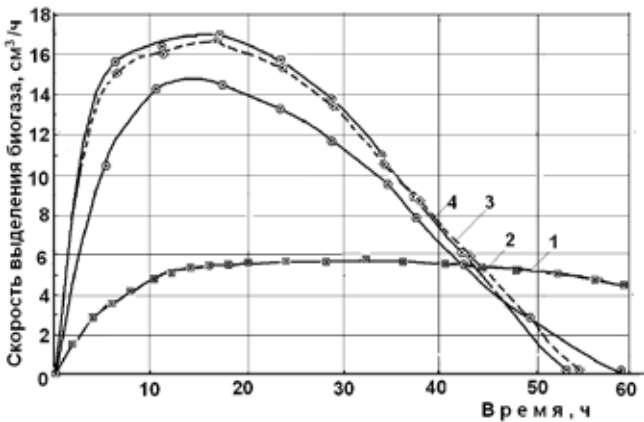
Рис. 1. Скорость выделения биогаза в условиях сбраживания с добавлением БВА (бетулинол + ама-рант в соотношении 1:1): 1 – контроль; 2 – 2,5 мг/л; 3 – 5,0 мг/л; 4 – 10,0 мг/л
