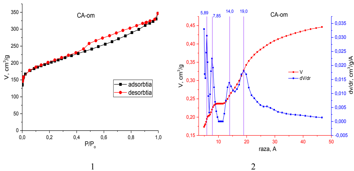
Figura 1. Izotermele de adsorbție și desorbție a azotului (77K) pe cărbunele activ din mangal de lemn (1) și curba de repartiție a porilor pe dimensiuni (2) pe cărbunele activ CA-om.
