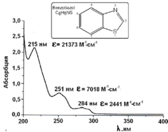
Рис. 2 Спектр в УФ-видимой области бензотиазола (ВТ) 0,1 моль в воде при pH=7,0
